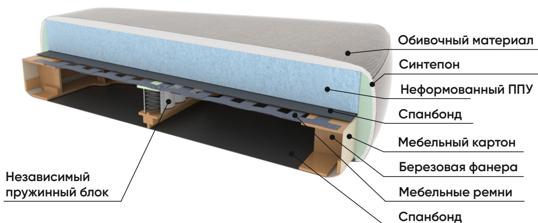
Рис.3 Разрез элемента
