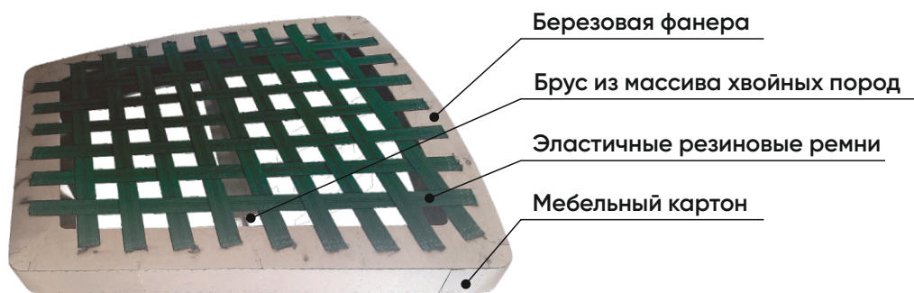
Рис.1 Каркас K23
